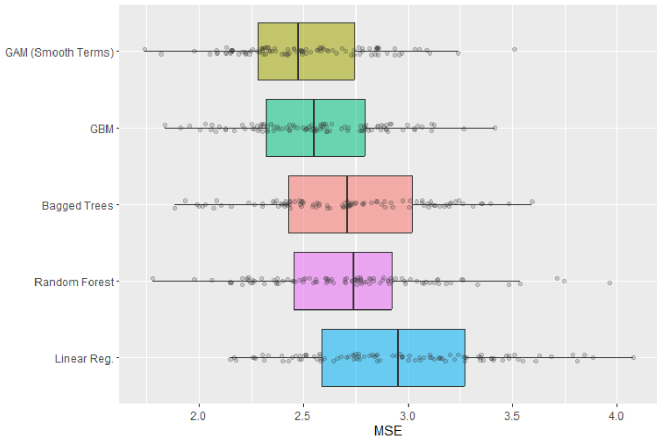
Рисунок 16 - Коробкова діаграма
