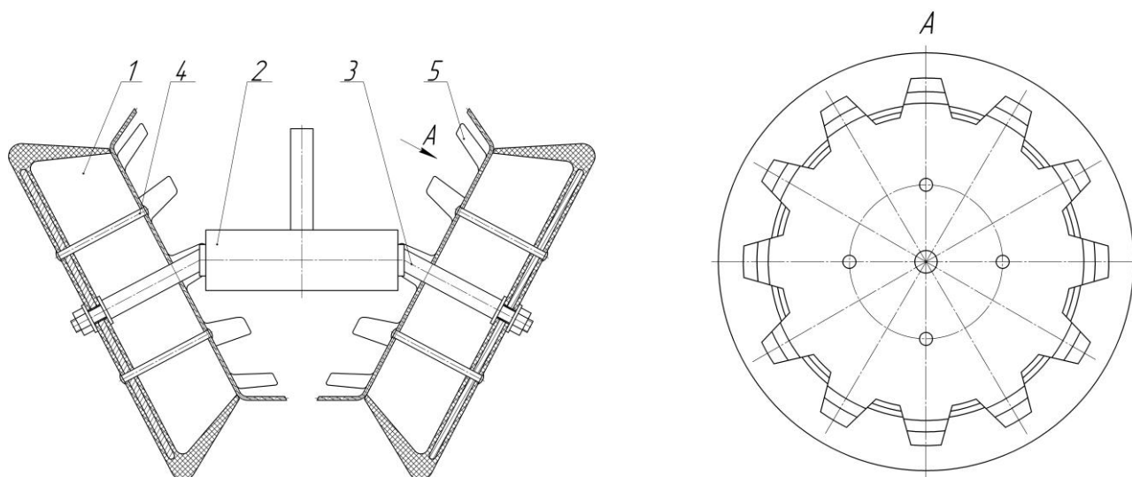
Рис. 1. Загортаючий робочий орган картоплесадильної машини:
