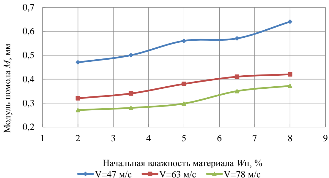
Рис. 5. Залежність модуля помола M від початкової вологості матеріала W_n .
