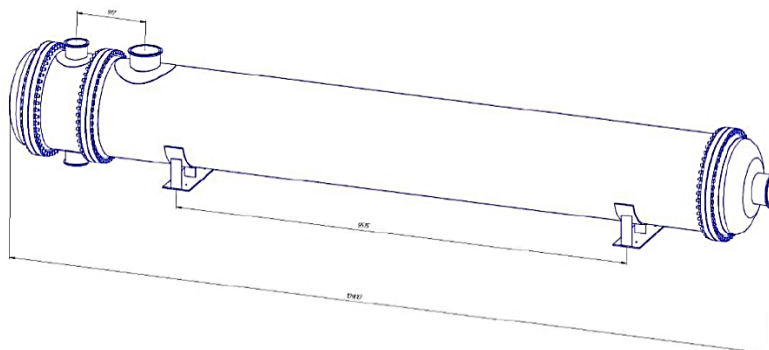
Рис. 2. 3D модель спроектованого кожухотрубчатого теплообмінника.
