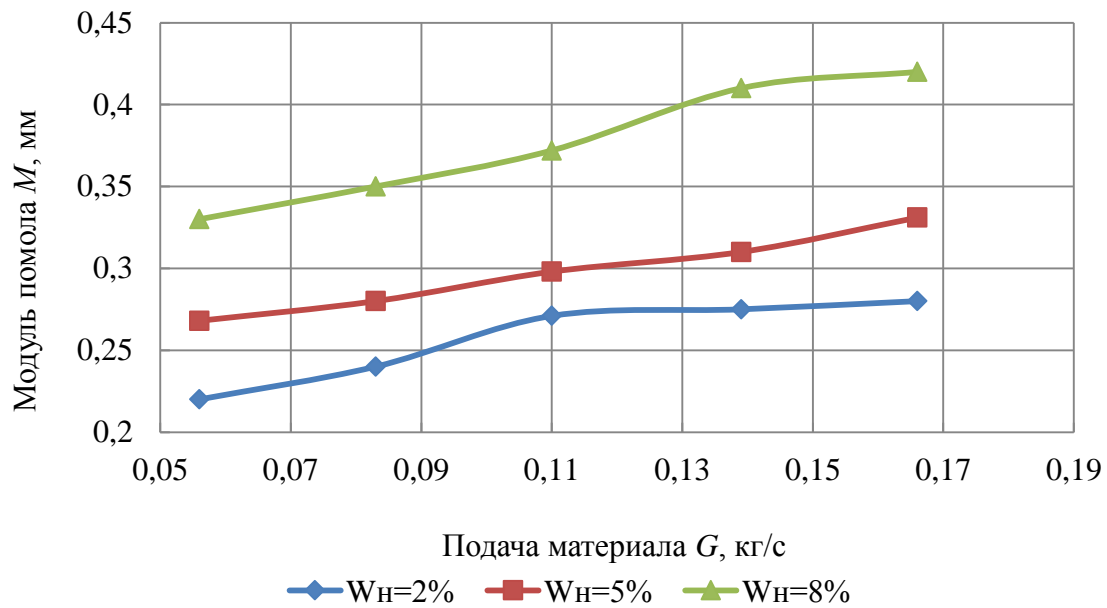
Рис. 4. Залежність модуля помола M від величини подачі матеріала G .
