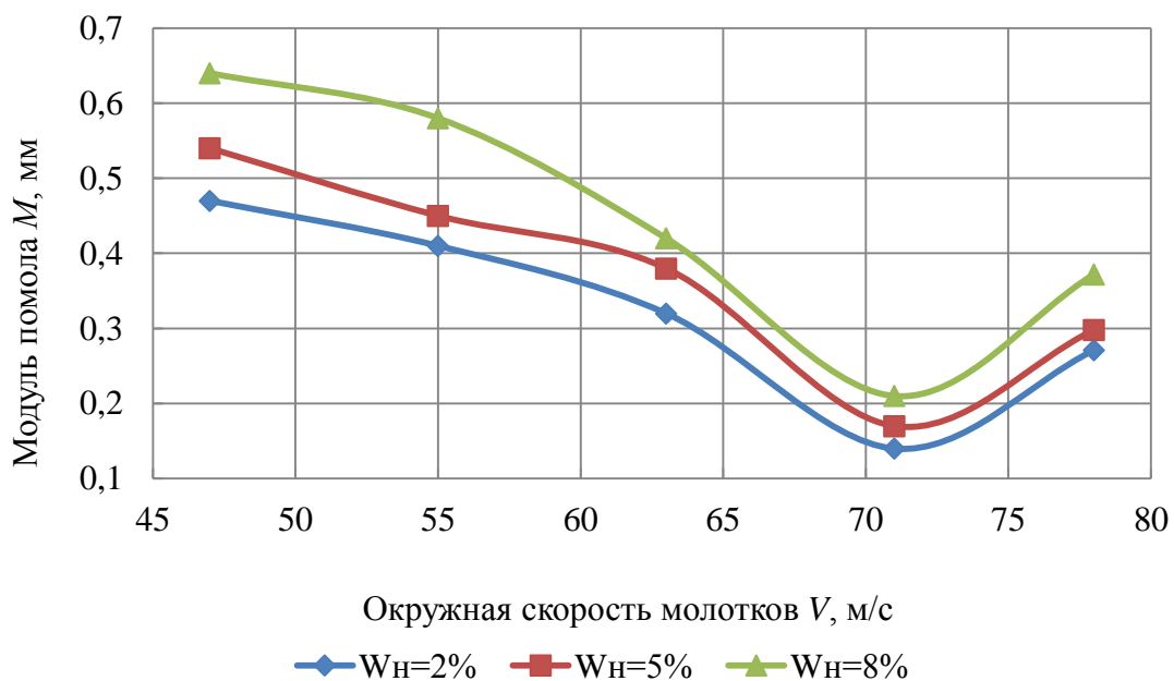
Рис. 2. Зависимость модуля помолу M от окружной скорости молотков V .
