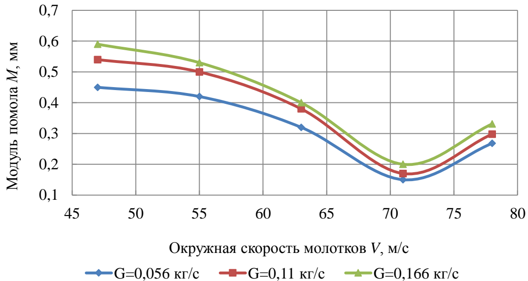
Рис. 1. Зависимость модуля помолу M от окружной скорости молотков V .
