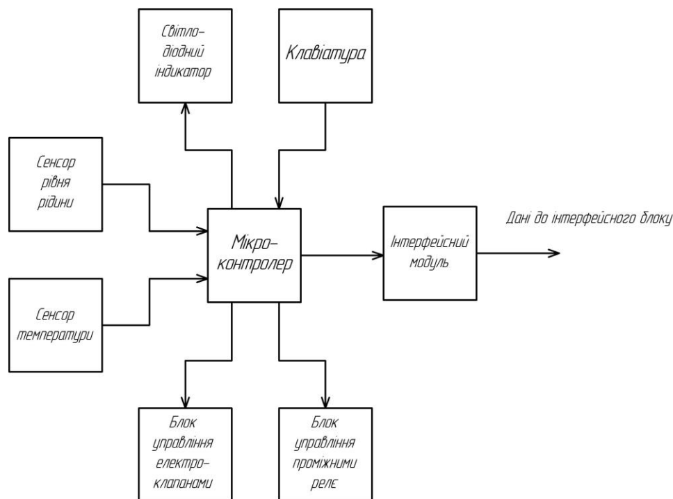
Рисунок 1 – Блок управління автоматом промивання. Схема електрична структурна.
